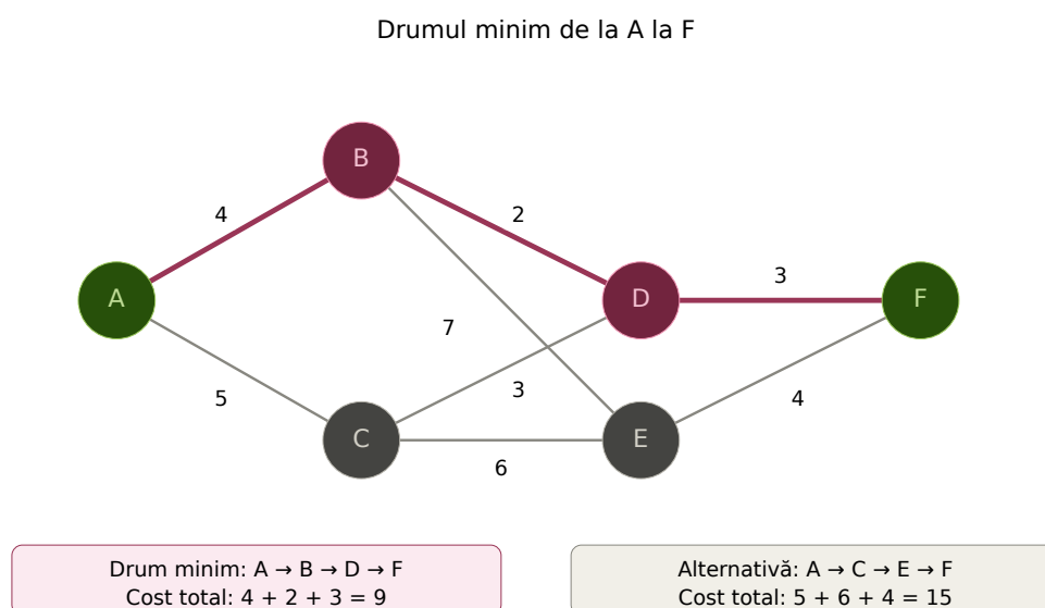
Figura 1.1: Exemplu de aplicare a algoritmului lui Dijkstra: drumul minim de la nodul A la nodul F este evidențiat cu roșu. Algoritmul găsește traseul A \rightarrow B \rightarrow D \rightarrow F cu cost total 9, în detrimentul alternativei mai lungi prin C și E (cost 15).
